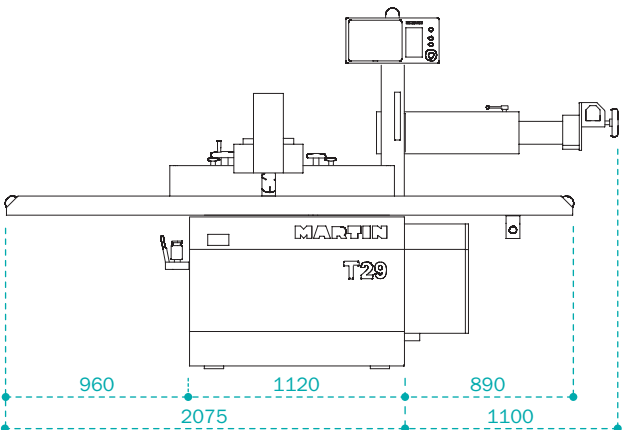
T29 con extensión de mesa | Vista frontal
