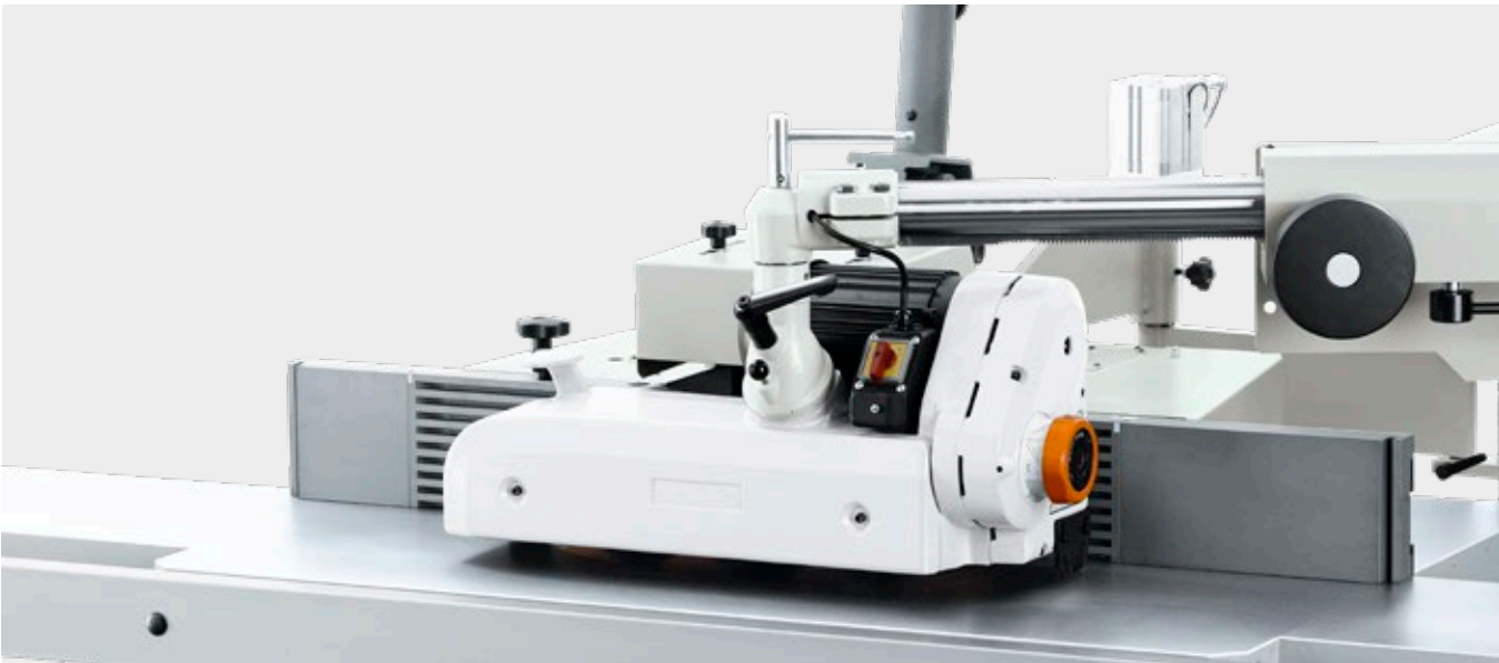
Avance Variomatic 4N en el soporte de avance | T2923_400+ T2915
