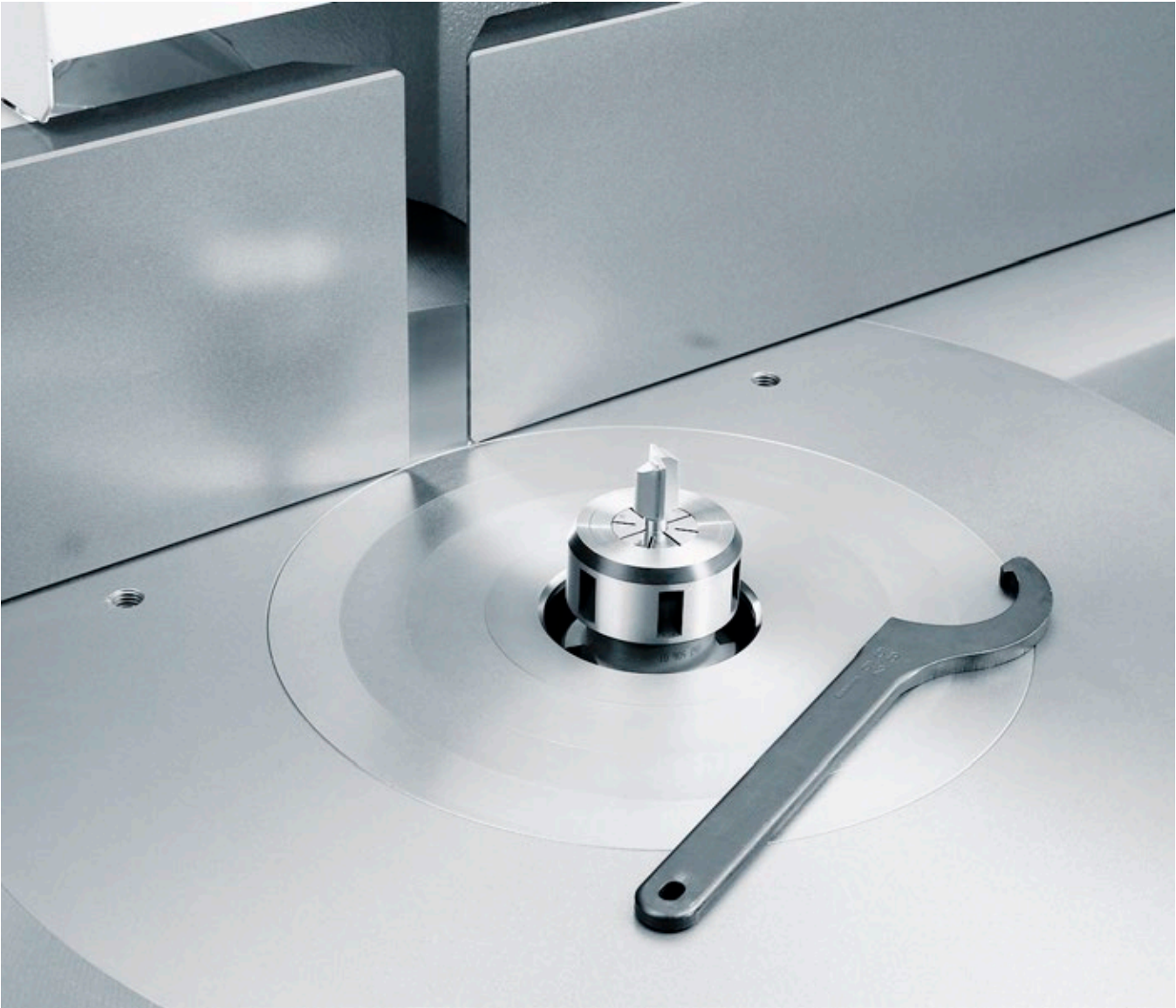
Mandril de pinza portapieza SK 40 | T2963
