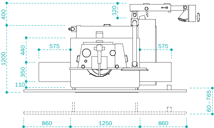
T29 con extensión de mesa | Vista superior
