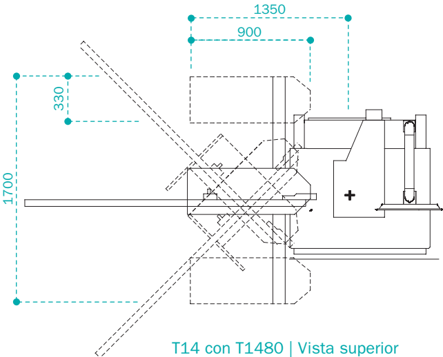
T14 con T1480 | Vista superior
