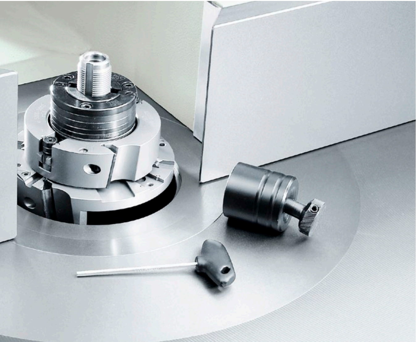
Sistema de sujeción rápida para mandril portafresa | Txx69
