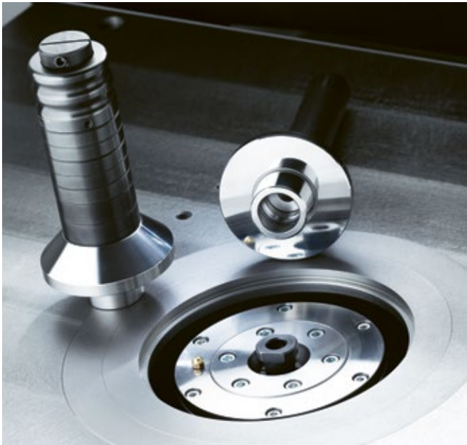
Sistema di serraggio del mandrino portafresa HSK 63 F | Txx70_63F
